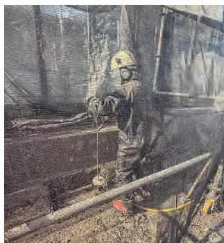
Betonsanierung unter Schutznetz.
